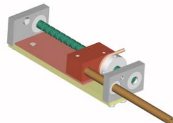
Actuator Assemblies
